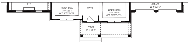
(ELEV. B)
